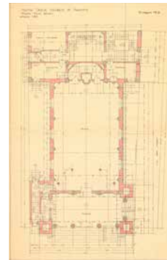
4. Tempio Valdese, Emilio Decker, planimetria piano terra scala 1:50, 1923. Archivio privato Tempio Valdese, Palermo.
