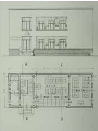
14. Salvatore Caronia Roberti, Casa provinciale delle Figlie di S. Anna in Villa delle Rose, progetto di ampliamento e sopraelevazione, corso Calatafimi, Palermo, 1939-1940. Alzato del prospetto e pianta del piano terra del padiglione scolastico maschile, riproduzione fotografica b/n in album fotografico (Archivio Fotografico, Fondo Caronia Roberti, Collezioni Scientifiche, Dipartimento di Architettura, Università degli Studi di Palermo)
