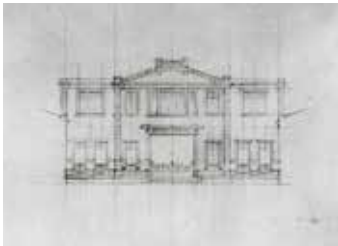
8. Ernesto Basile, Dispensario Polivalente e Sanatorio Diurno della Croce Rossa, prolungamento di via Lincoln (via Giorgio Arcoleo), Palermo, 1920-1928, alzato del prospetto del corpo centrale dell'edificio principale, terza variante, 1/100, matita su carta Fabriano, 484x664 mm, s.d., s.t. Nel verso: annotazioni a matita (Archivio Disegni, Dotazione Basile, Collezioni Scientifiche, Dipartimento di Architettura, Università degli Studi di Palermo)
