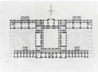
3. Ernesto Basile, Sanatorio Popolare per i Tubercolosi in Palermo, (1899), pianta del piano terra, variante, 1/200, china e matita su carta da lucido, 580x785 mm, s.d., s.t., firmato E. Basile; orientamento a china (Archivio Disegni, Dotazione Basile, Collezioni Scientifiche, Dipartimento di Architettura, Università degli Studi di Palermo)
